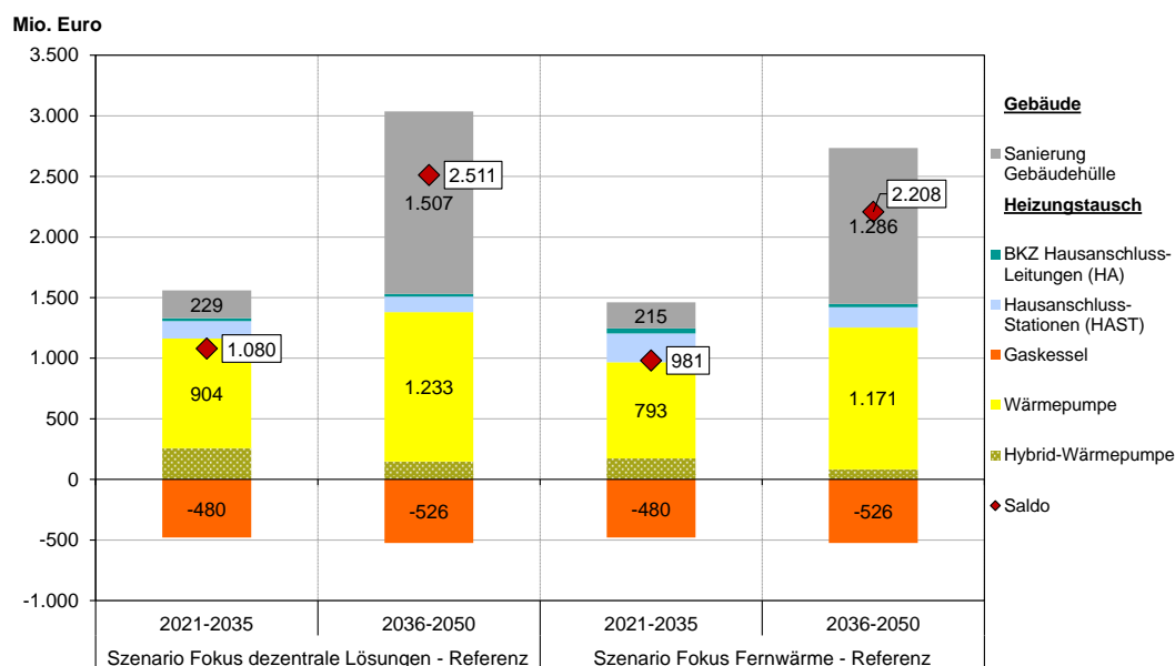
Abbildung 14-8 Kumulierte Investitionen in den zielorientierten Szenarien aus Sicht der Nutzenden (nach Förderung; inkl. MwSt.) im Vergleich zum Referenzszenario (negative Werte sind Einsparungen gegenüber der Referenz)
