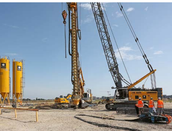
Bohrmaschine am Werk: Die Arbeiten am künftigen U-Bahnhof Freiham Zentrum beginnen.
