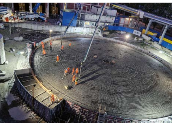
Das Fundament des künftigen Wärmespeichers der SWM am Standort Süd
